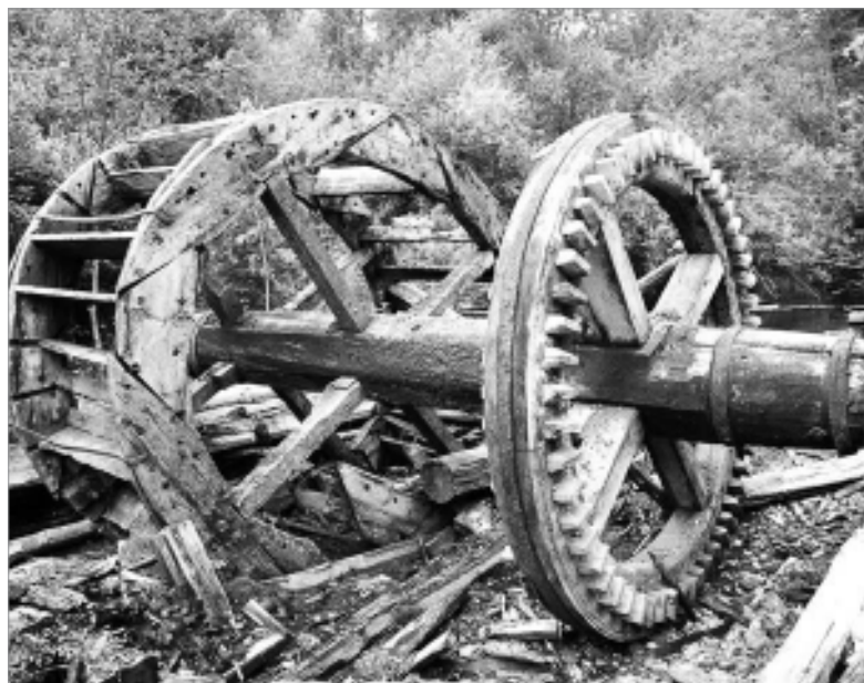
Остатки водяного колеса с зубчатым приводом
